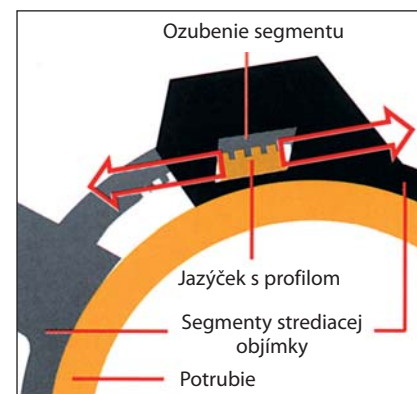
Obr. 2 Priechy rez
